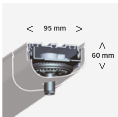
Dimensions du capot
